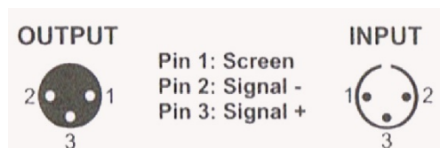
Conector DMX512 de três pinos (Canon)
